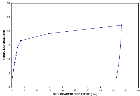
Figura 5 -Curva atrito lateral versus deslocamento do fuste (estaca 2).
