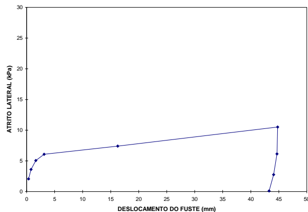
Figura 6 -Curva atrito lateral versus deslocamento do fuste (estaca 3).
